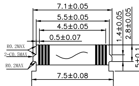
S1/S2端冲边图
